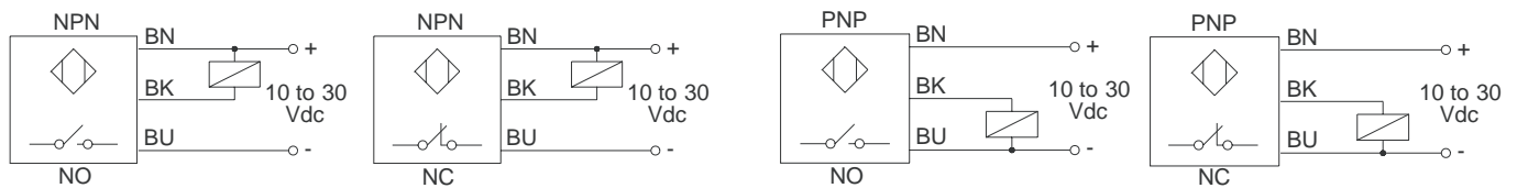
MQP2-1504(N/P)-(A/B)3U2F
